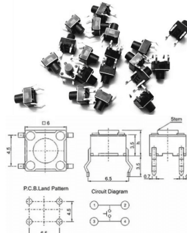
Pulsador 6 X 6 X 7mm Na Dip-4 Serie Tc-6615
