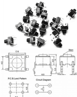
Pulsador 6 X 6 X 9.5mm Na Dip-4 Serie Tc-6615
