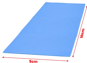
Almohadilla Térmica De Silicona, Thermal Pads 6.0w/m-k 10x5cm 0.5mm
